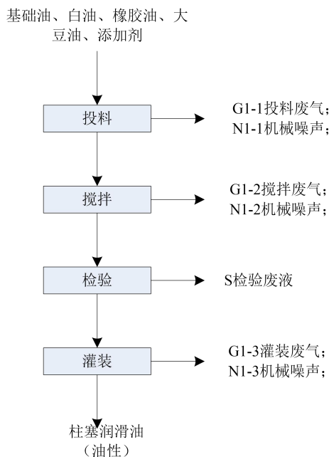
图2-2 柱塞润滑油（油性）工艺流程图
