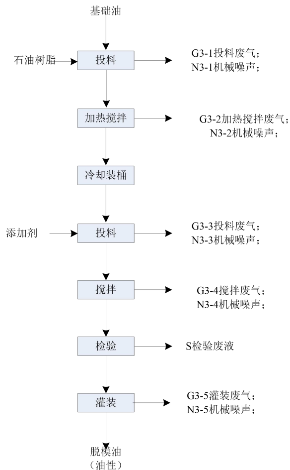
图2-3 脱模油（油性）工艺流程图
