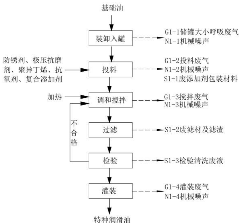
图2-2 特种润滑油工艺流程图
