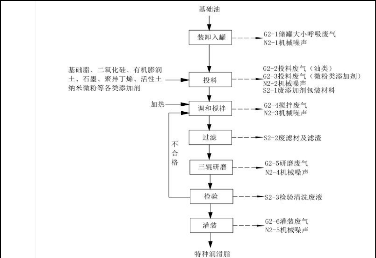
图2-3 特种润滑脂工艺流程图
