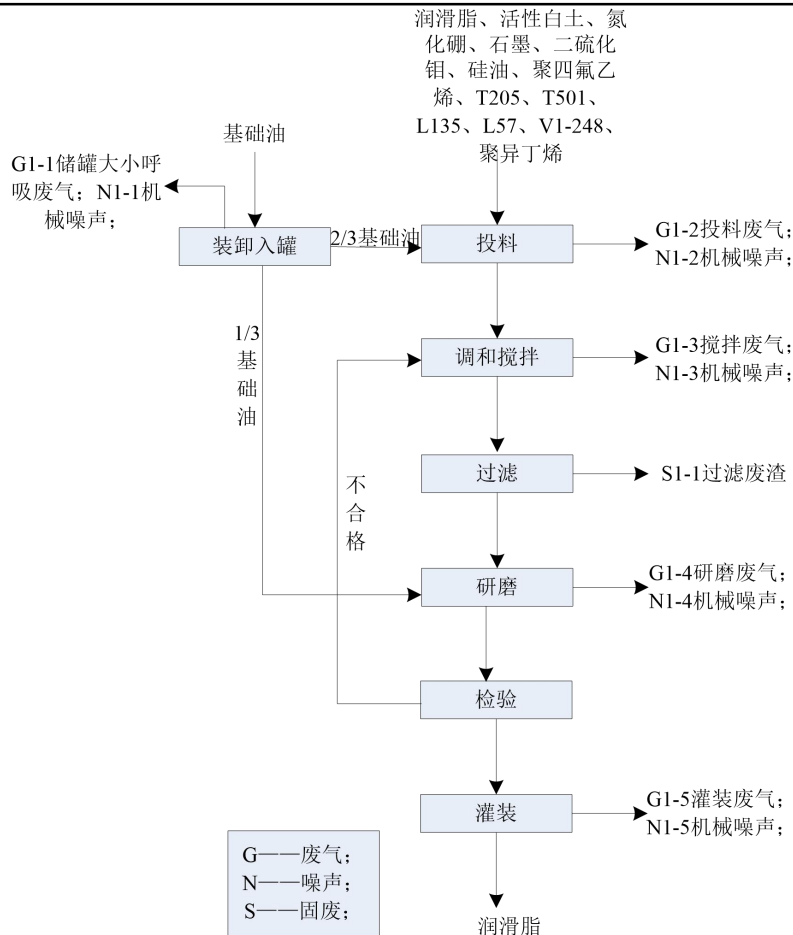
图2-2 润滑脂工艺流程图
