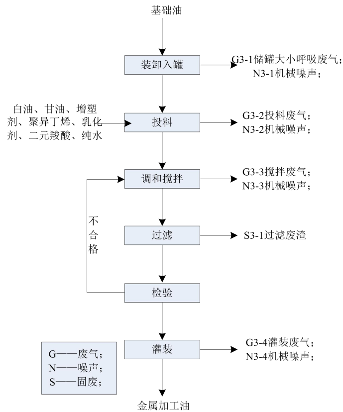
图2-3 金属加工油工艺流程图
