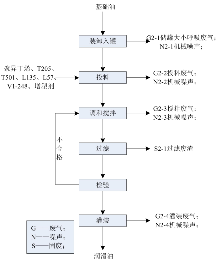
图2-3 润滑油工艺流程图
